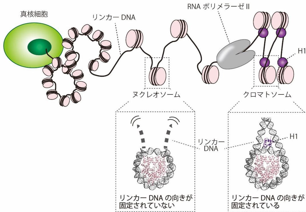
図1. 真核生物の DNA 折りたたみ構造のイメージ図
