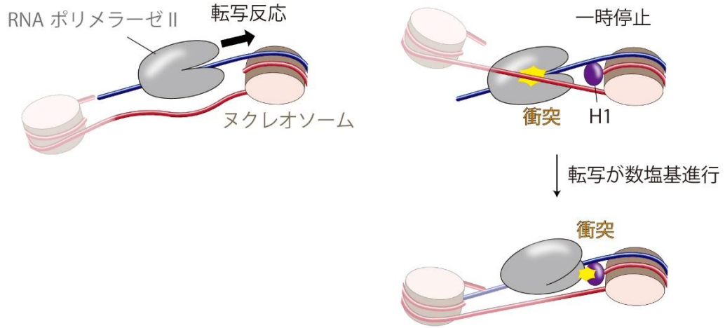
図3. 本研究から得られた、RNA ポリメラーゼ II が H1 により折りたたまれた DNA を転写するモデル図
