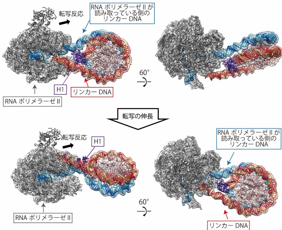
図2. 本研究で明らかになった、H1 が RNA ポリメラーゼ II をヌクレオソームの手前で一時停止させる各ステップの構造
